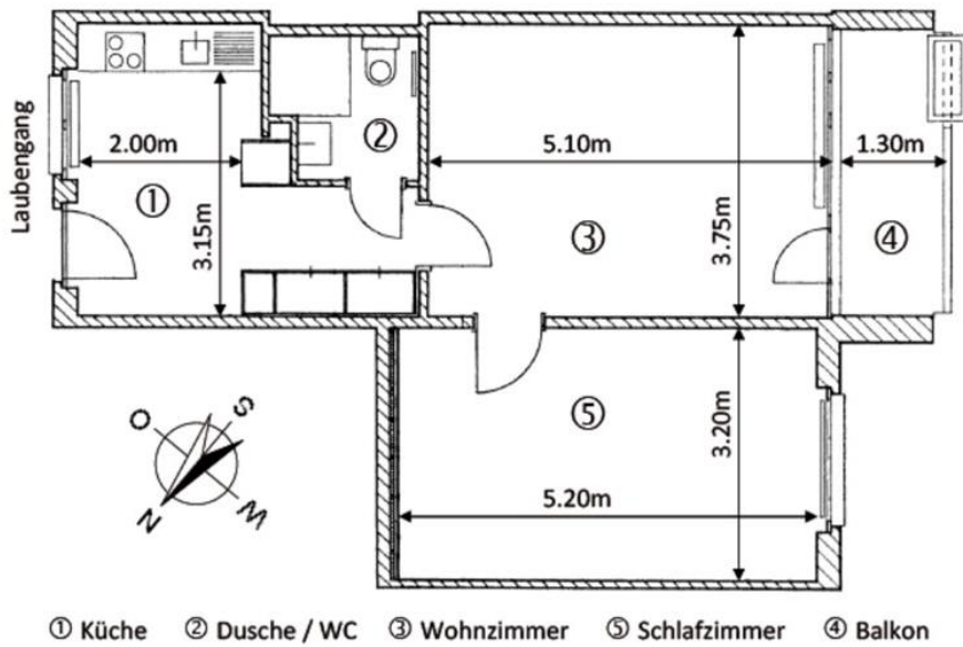
Zweizimmer-Wohnung (35m 2 ), Kellerabteil 6.4m 2
